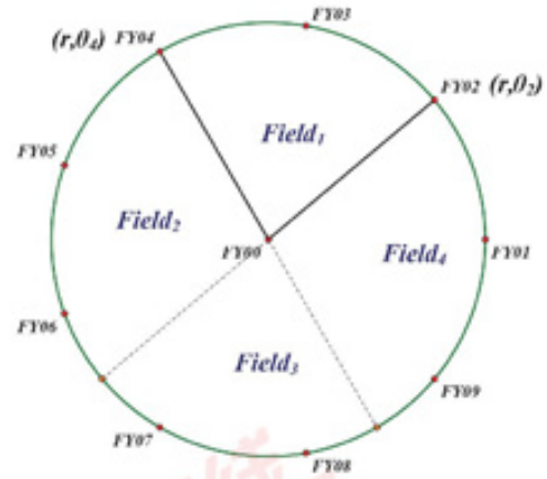
图 3: 正弦定理求解坐标的局限性
